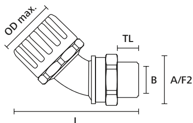
HeliaGuard fittings, 45° med omløber, udvendig gevind
