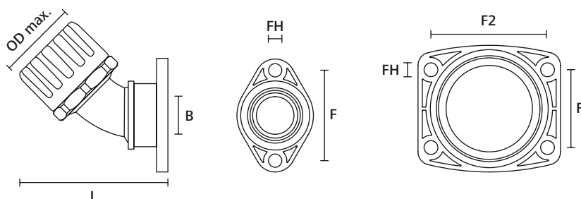
HeliaGuard fittings, 45° omløber flange
