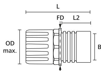
HeliaGuard fittings, reduktionsstykke
