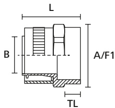
Helaguard fittings, lige med fast indvendig gevind
