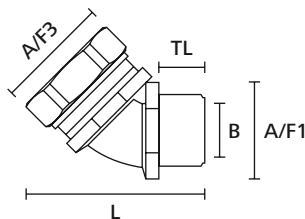
HelaGuard fittings, 45° med fast udvendig gevind
