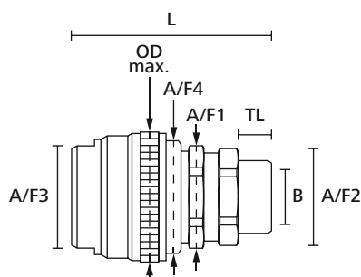
HeliaGuard fittings, lige med omløber udvendig gevind
