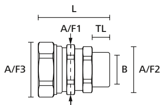
HelaGuard fittings, lige med omløber udvendig gevind
