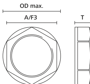
HelaGuard låsemøtrik
