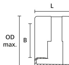
HelaGuard afslutningshætte
