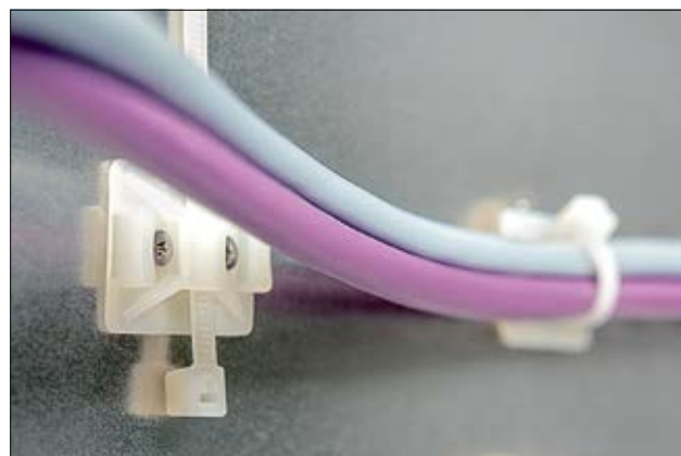
Mocowania serii TY o prostokątnym przekroju.
