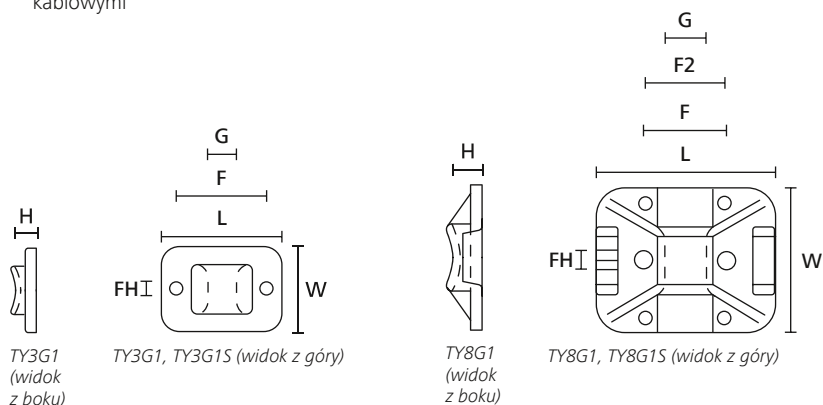
Mocowania serii TY o prostokątnym przekroju.
