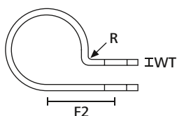
Obejma Alu P-Clip (widok z boku)
