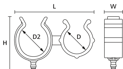
Uchwyt DTC do rury (widok z przodu)
