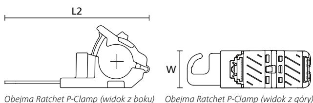
Obejma Ratchet P-Clamp (widok z boku) Obejma Ratchet P-Clamp (widok z góry)
