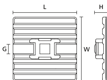
Elastyczny, samoprzylepny element mocujący FMB4APT-I (widok z góry)
