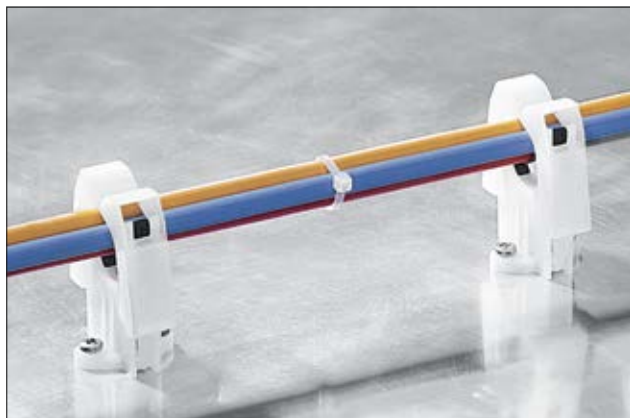
Wspornik wiązki HH20 do stołów montażowych.
