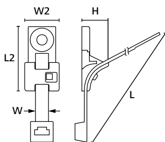
HDM z opaską kablową (L= długość opaski kablowej)
