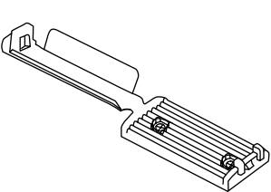
Mocowanie odbywa się za pomocą wkrętów M3 lub akrylowej taśmy klejącej.
