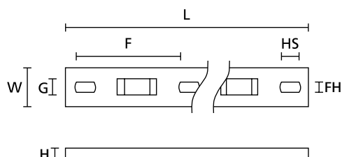
Listwy mocujące MP i MSMP (widok z góry i z boku)
