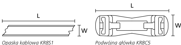
Opaska kablowa KR8S1
