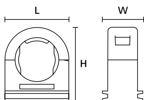
Uchwyt HelaGuard (widok z boku)
