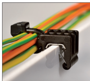
T50ROSEC23, de bundel wordt parallel aan de rand geleid.
