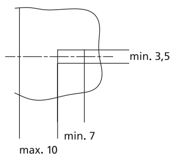
Positie van het boorgat van de extra lip
