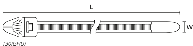
Opaski z mocowaniem kotwicznym tego typu umożliwiają stosowanie w obszarach o ograniczonej przestrzeni.
