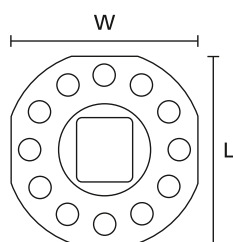
Cokół PMB5 (widok z góry)
