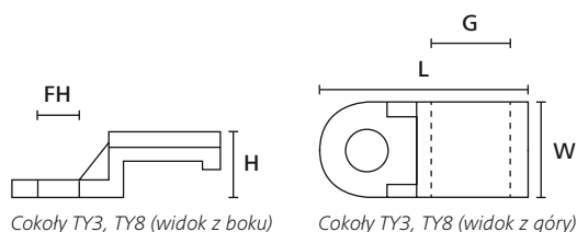
Cokoły TY3, TY8 (widok z boku)
