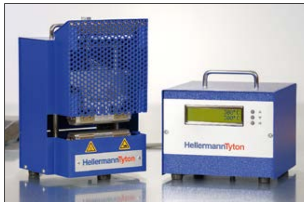
Urządzenie do szybkiego obkurczania termokurczy ShrinkPad 110 składa się z jednostki sterującej, prasy obkurczającej, przewodu sieciowego oraz łącznika nożnego.
