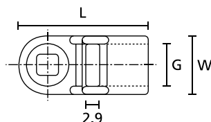
Cable tie base SBH1,3
