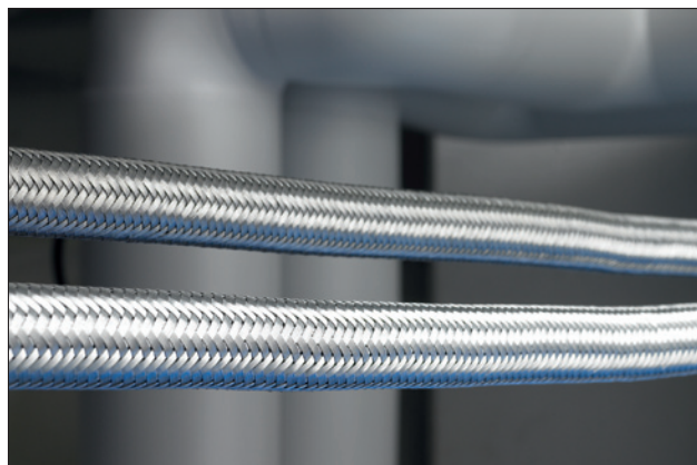
HelaGuard PCSB, Galvaniserad stålslang med PVC överdrag samt ett extra överdrag av galvaniserad flätad stålstrumpa. Ger hög resistens mot nötning och EMC skärmning.
