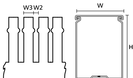
HTWD-PN-johdotuskouru
