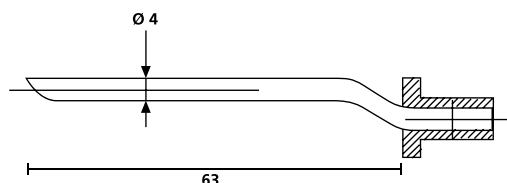
8-laajennuskärki
