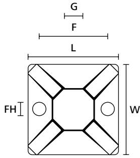
MB3-MB5 (üstten görünümü)
