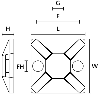
MCMB Montajı (yandan ve üstten görünüm)
