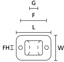
TY3G1, TY3G1S (üstten görünümü)
