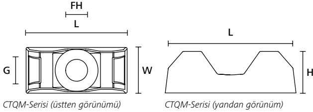
CTQM-Serisi (üstten görünümü)
