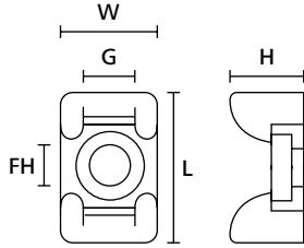
KR6G5, KR8G5 ve CTM (üstten görünümü)
