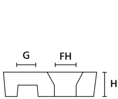
MB1, MB2 Kroşeleri (yandan görünüm)
