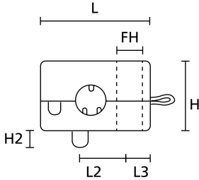
Klam-Klip (yandan görünüm)
