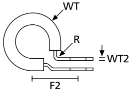
Kloropren uçlu ALU_C P-Kelepçe (yandan görünüm)
