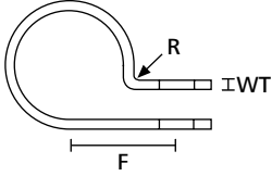
P-Kelepçe H1P - H18P (yandan görünüm)
