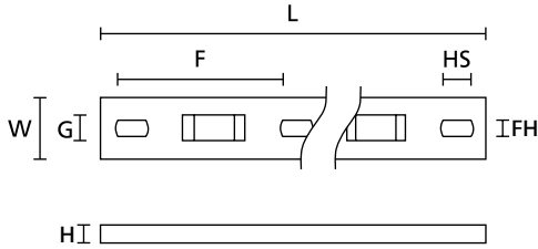
MP ve MSMP Tipi Montaj kroşeleri
