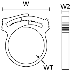
SNP - Kilitli Hortum Klipsleri
