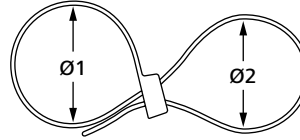
DH-Serisi maksimum kombine demet çapı
