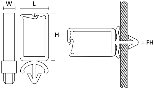
WPC Kablo İtmeli Klips (yandan görünüm, önden görünüm, uygulamada)
