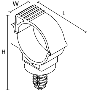
Yalnızca boyutlar için referans çizim
