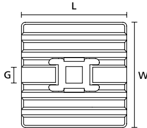
Esnek Yapışkanlı Montaj FMB4APT-A (üstten görünümü)
