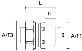
HelaGuard sıkıştırma fittingi, sabit dış dişli ile düz
